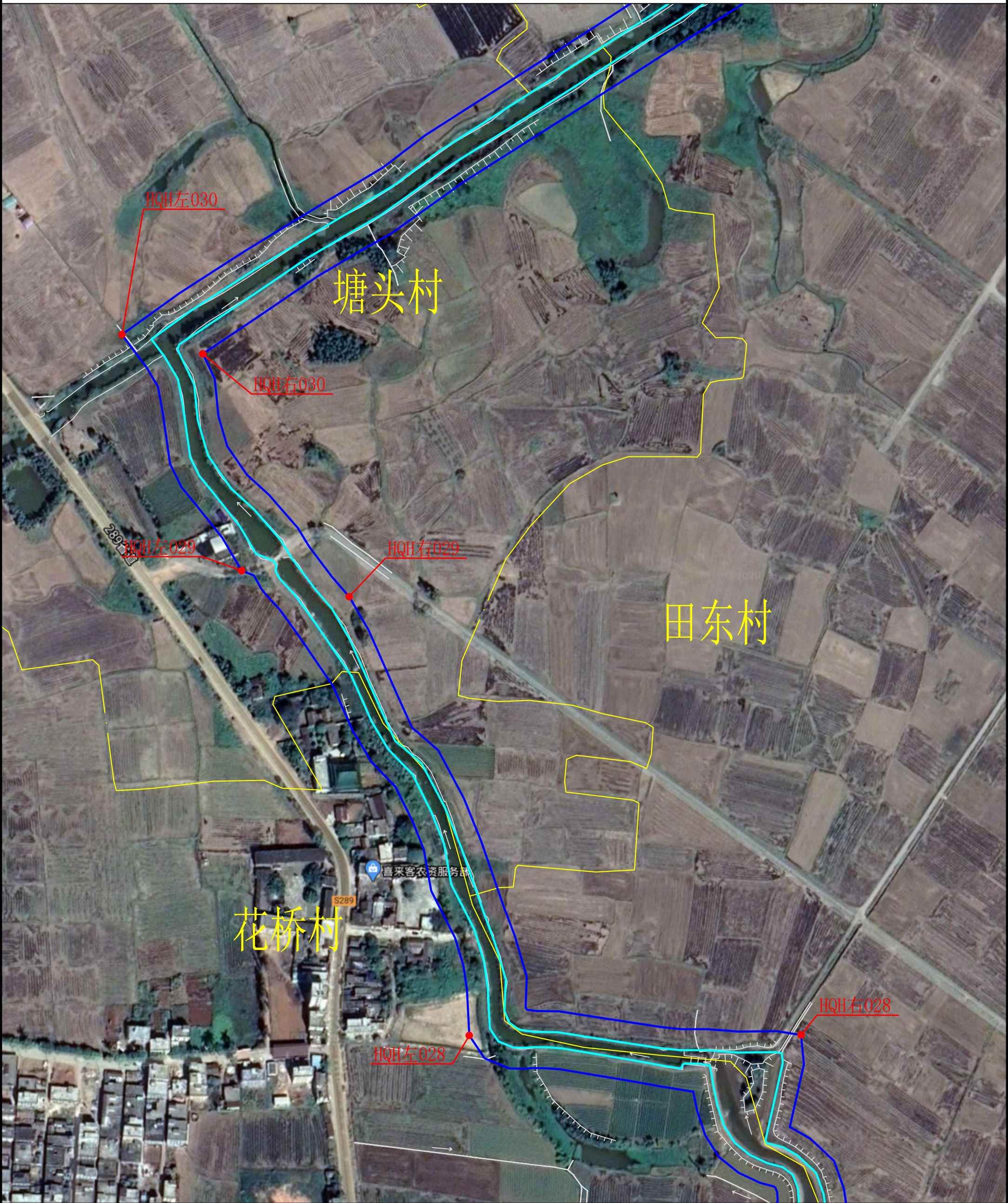
雷州市花桥河河道管理范围线平面图(14/27)
